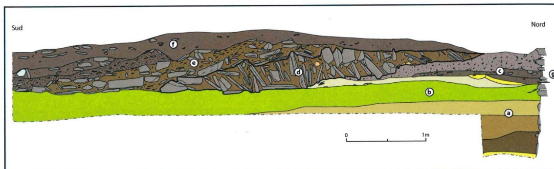
Fig. 2. Coupe de l'effondrement du pignon sud : (a) sol en place, (b) limon perturbé, (c) couches d'occupation et remblais, (d) mur effondré, (e) pierres «remuées», (f) couche supérieure, (g) mur sud en place. Dessin J.-F. Baltus, H. Jacques et J. Roland, infographie J.-F. Baltus © ARC-HAB.
